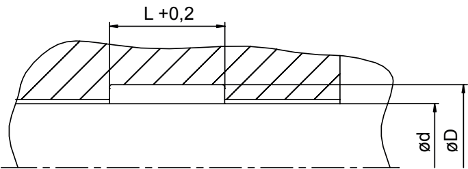
Fig. 5, Rod guide ring
